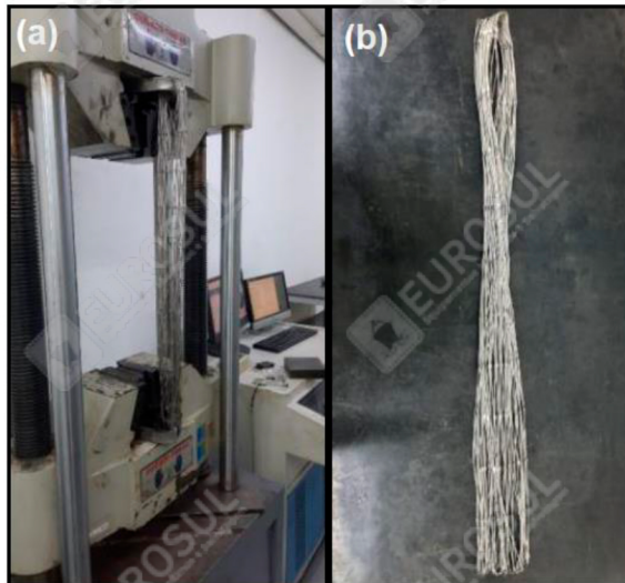
Figura 2 – Amostra (a) durante e (b) após o ensaio de Tração.
